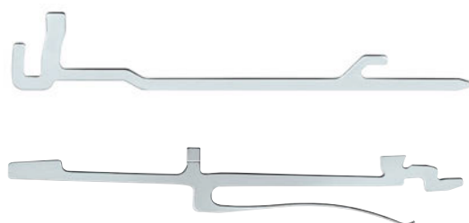
选针片 (AT/ATF)
